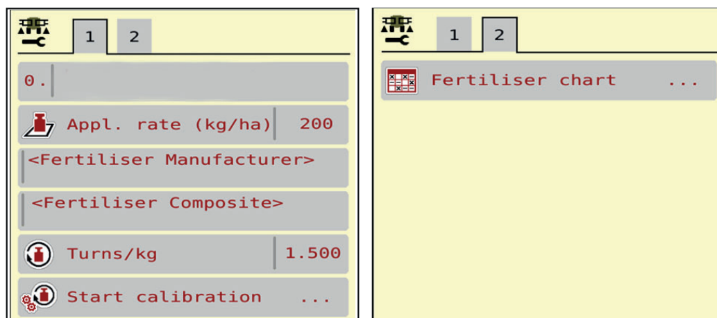
图 4.3: 肥料设置菜单标签页 1 和 2
