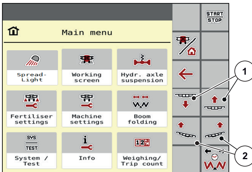
图 4.13: 功能键悬臂倾斜度 / 高度调整
