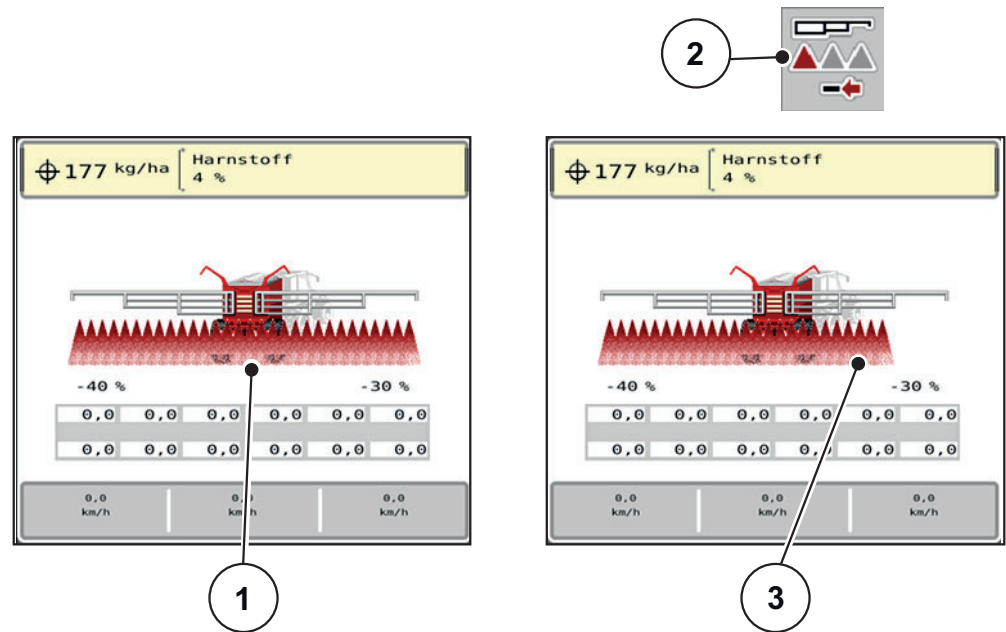
图 2.4: 部分宽度状态的显示
